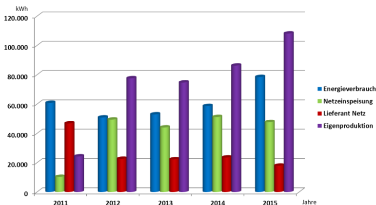
© Autoservice-Demmler, Energieerzeugung/ Eigenverbrauch im Unternehmen
