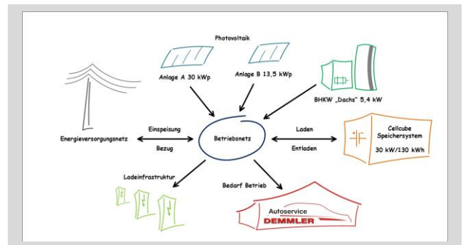
Energiemanagementansicht – intelligentes Betriebsnetz © Autoservice- Demmler
